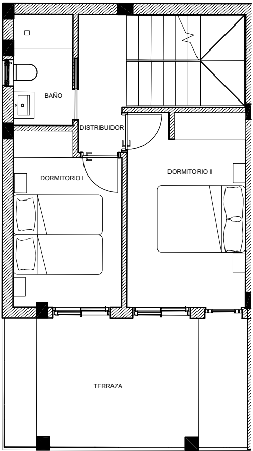
PLANTA -1 (NOCHE)
