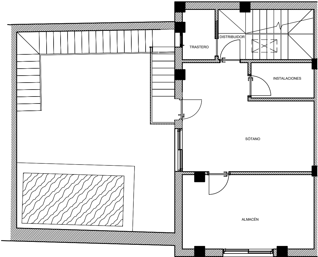
PLANTA SEMISÓTANO
